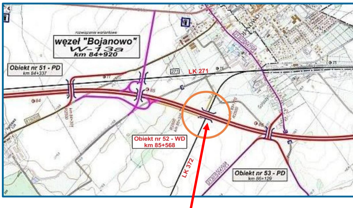
Wiadukt kolejowy nad drogą S5
